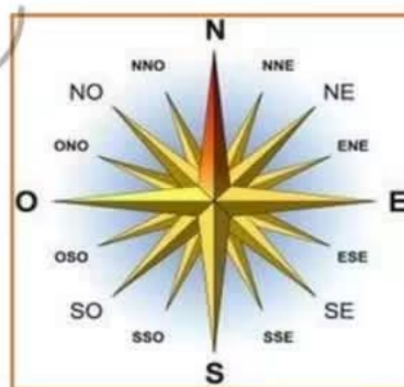
Fig. 4 : Principales orientations des cartes topographiques
