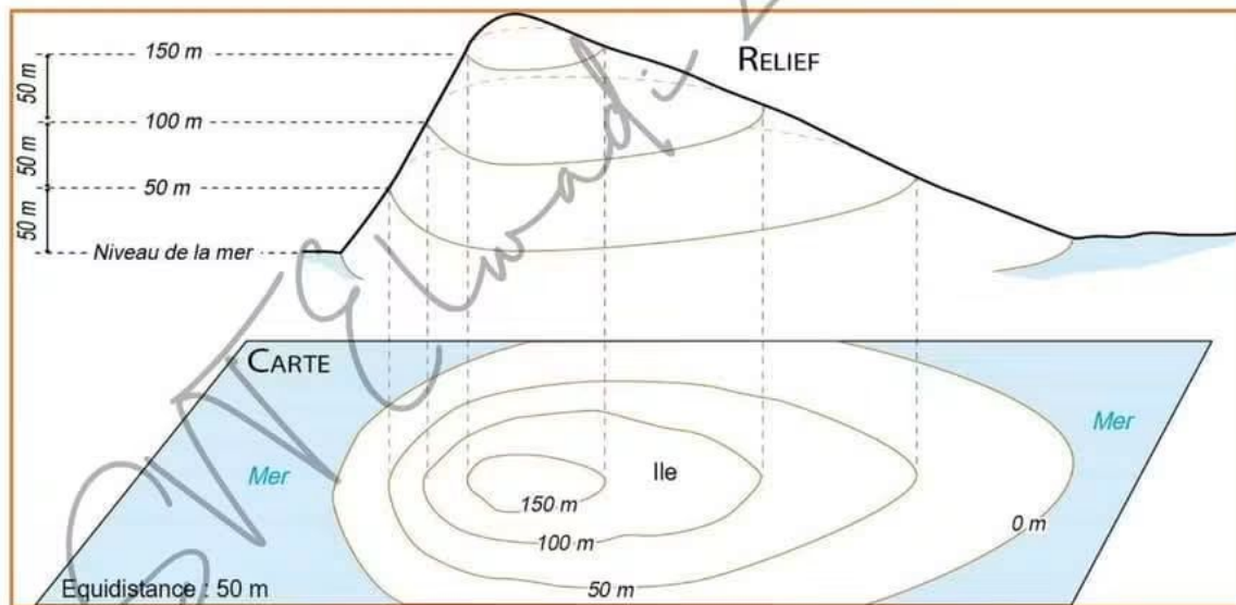
Fig. 1 : Principe d'établissement des courbes de niveaux
